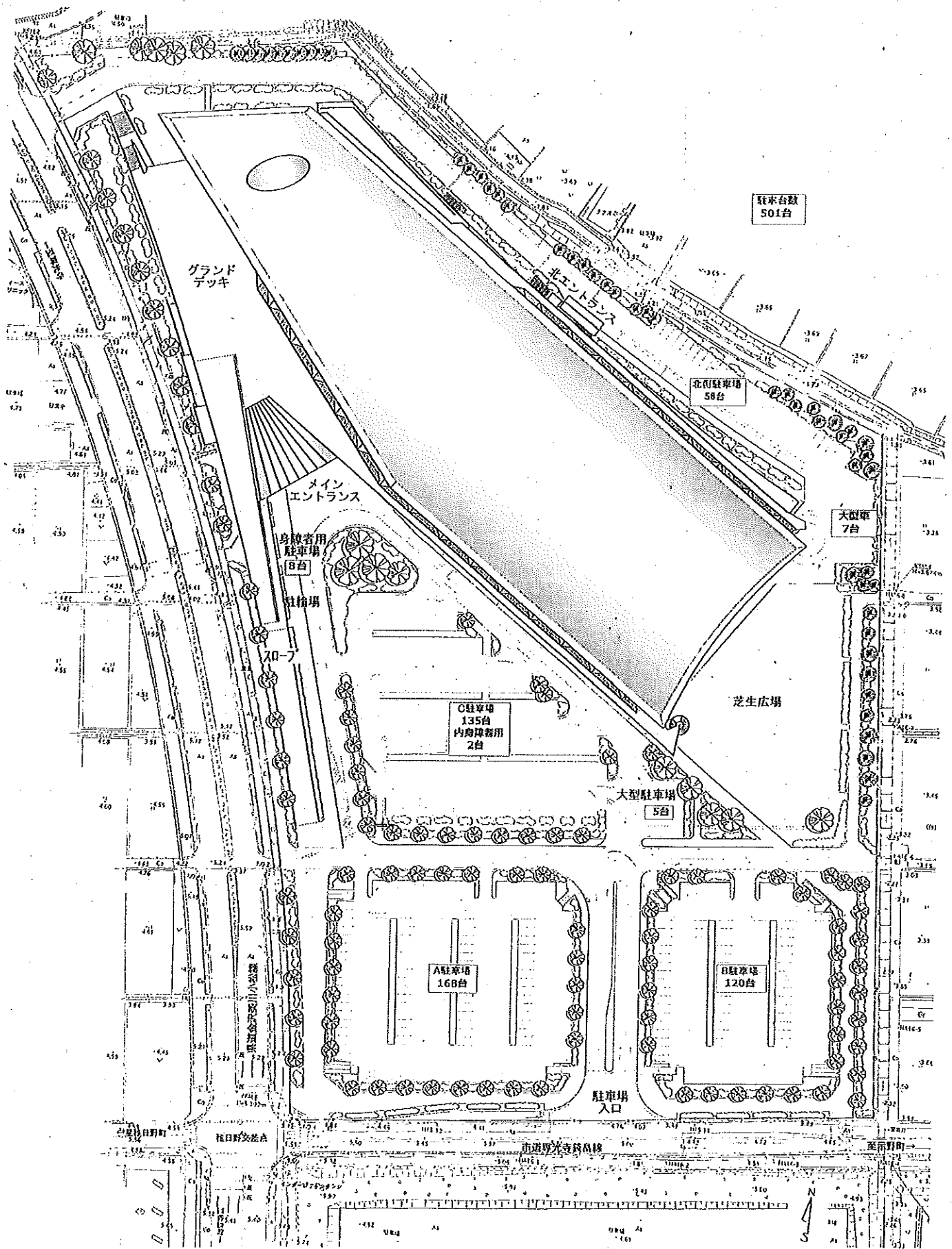
配置図 S : 1/700
